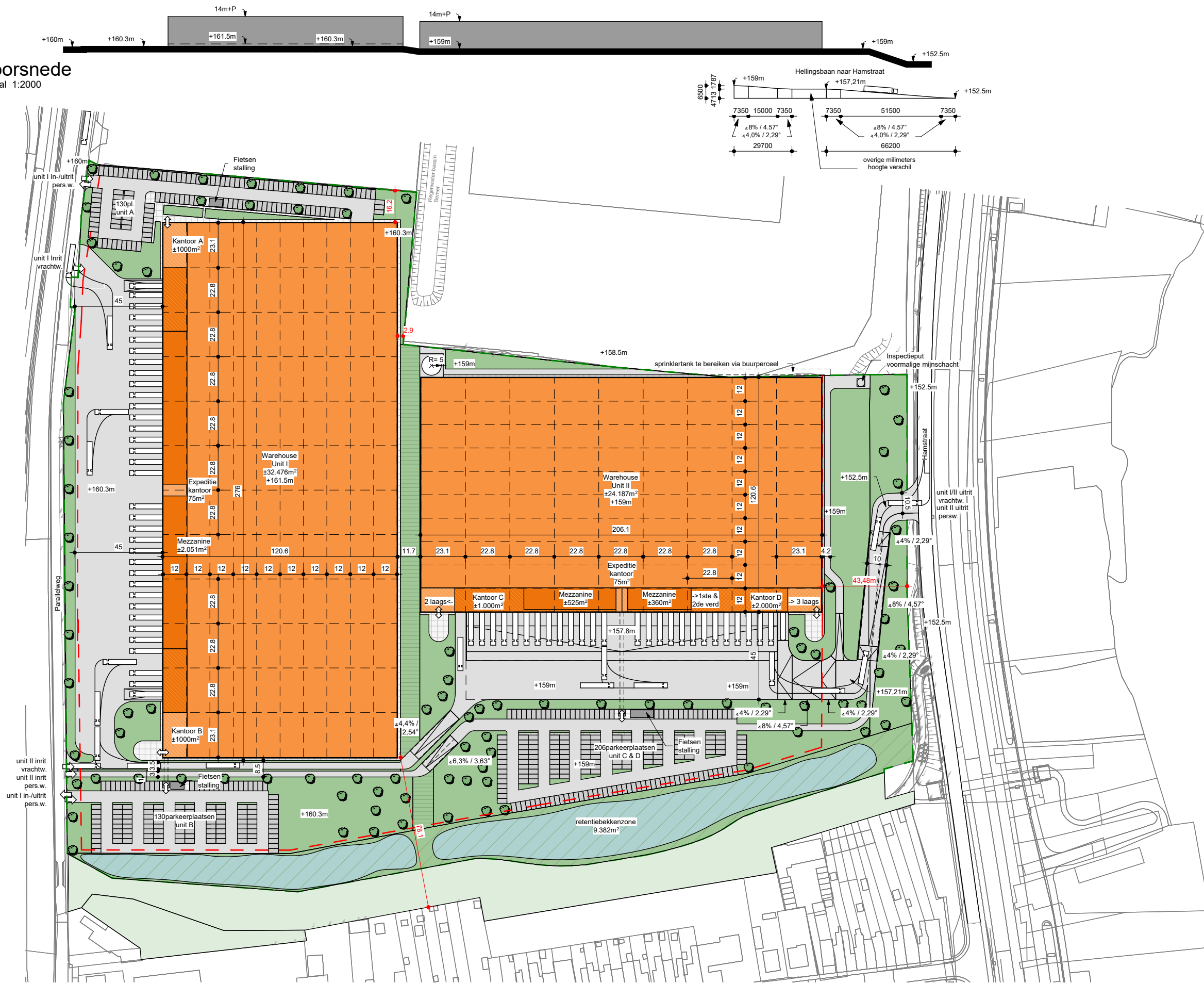
Overzichtstekening terrein schaal 1 : 2000
